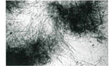
チロシン*
