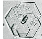
シスチン*
